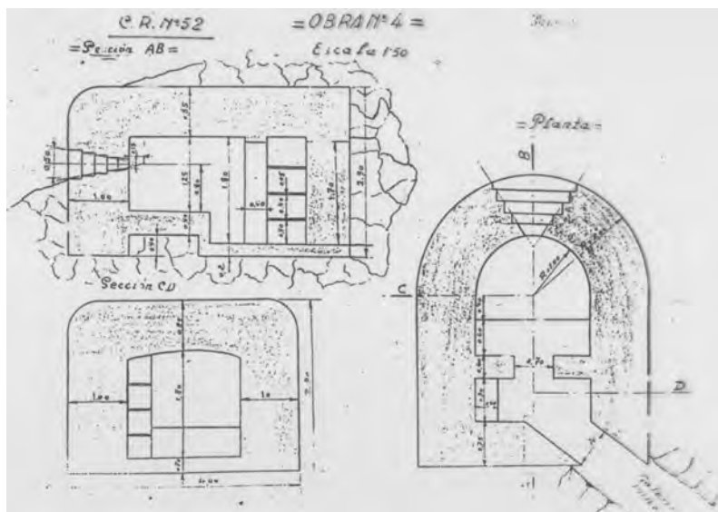
Secció de la construcció d'un búnquer
